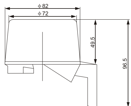
Exterior dimension(mm)
